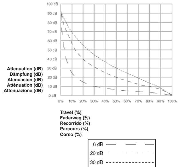
Channel Slide Curve Kanalfaderkurve Curva de los mandos deslizantes de canal Courbe des curseurs de canal Curva cursori canale
